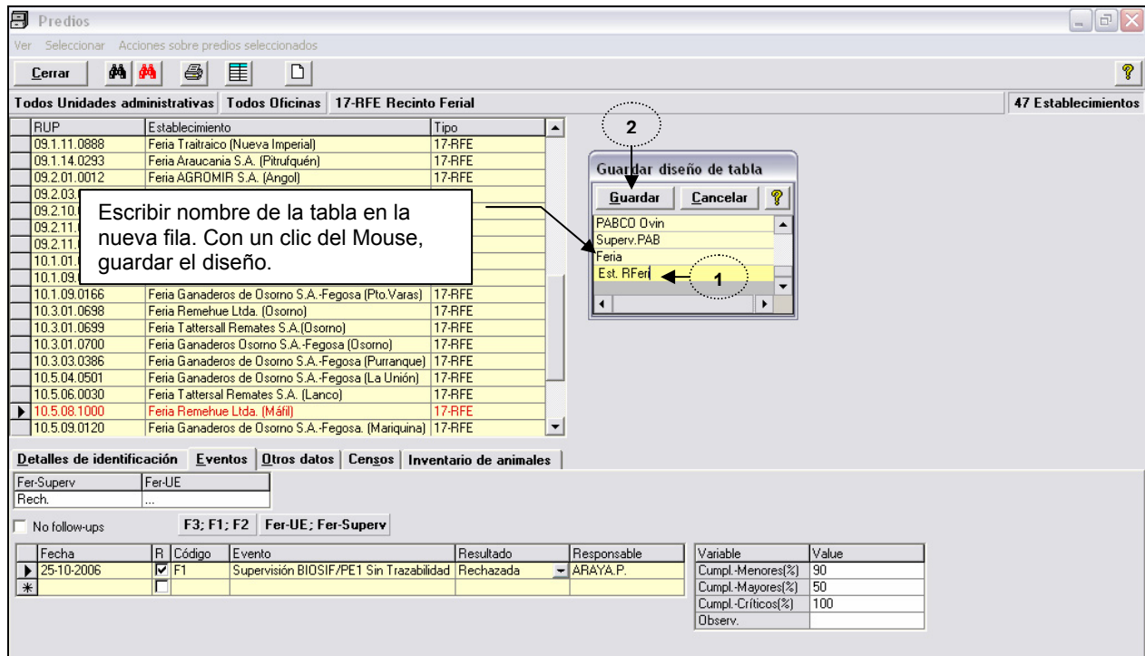
Fig. 10 Nombrar diseño de tabla para recintos feriales.
