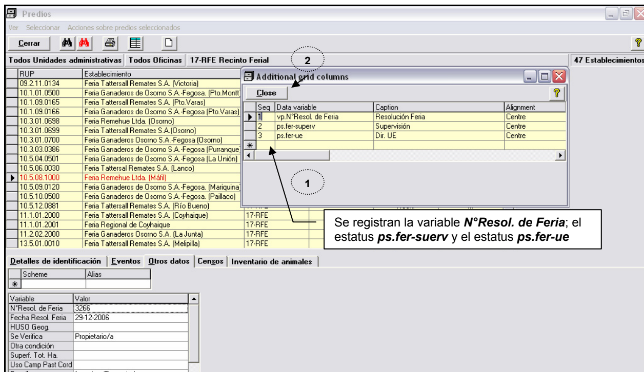
Fig. 15 Incorporación de columnas para indicar el número de resolución, el resultado de la última supervisión y si está o no en el directorio UE para recintos feriales con trazabilidad individual.
