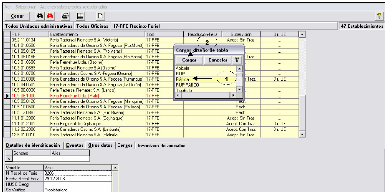
Fig. 18 Cargar diseño de tabla.
