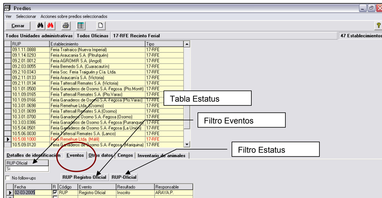
Fig. 4 Carpeta Eventos. Lugar donde se registran los eventos del establecimiento seleccionado. En esta carpeta se visualizan los eventos y estatus del establecimiento.
